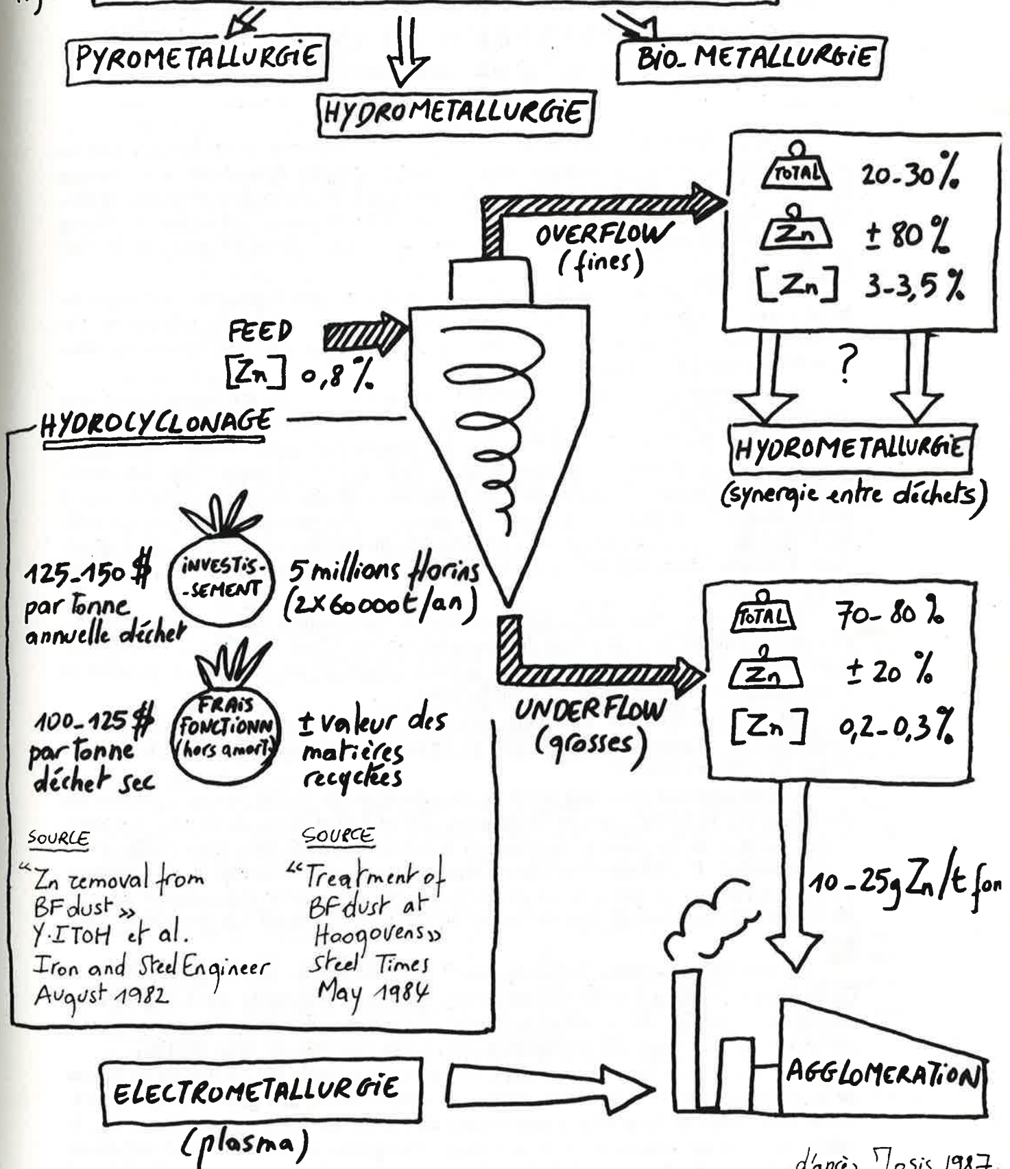
Fig.5. RECYCLAGE DES BOUES DE HAUTS FOURNEAUX
